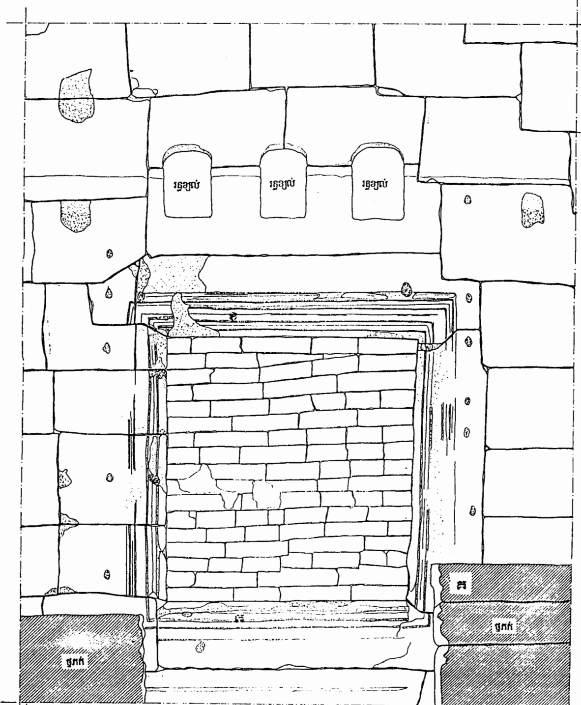
រូបភាពកំពស់មើលពីខាងក្រៅ
