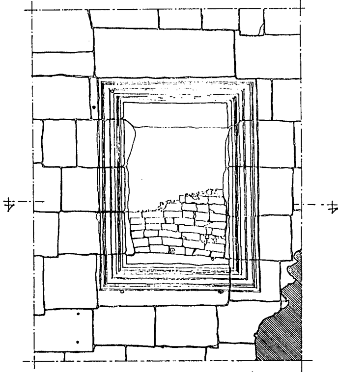
រូបគោតកំពស់មើលពីខាងក្រៅ
