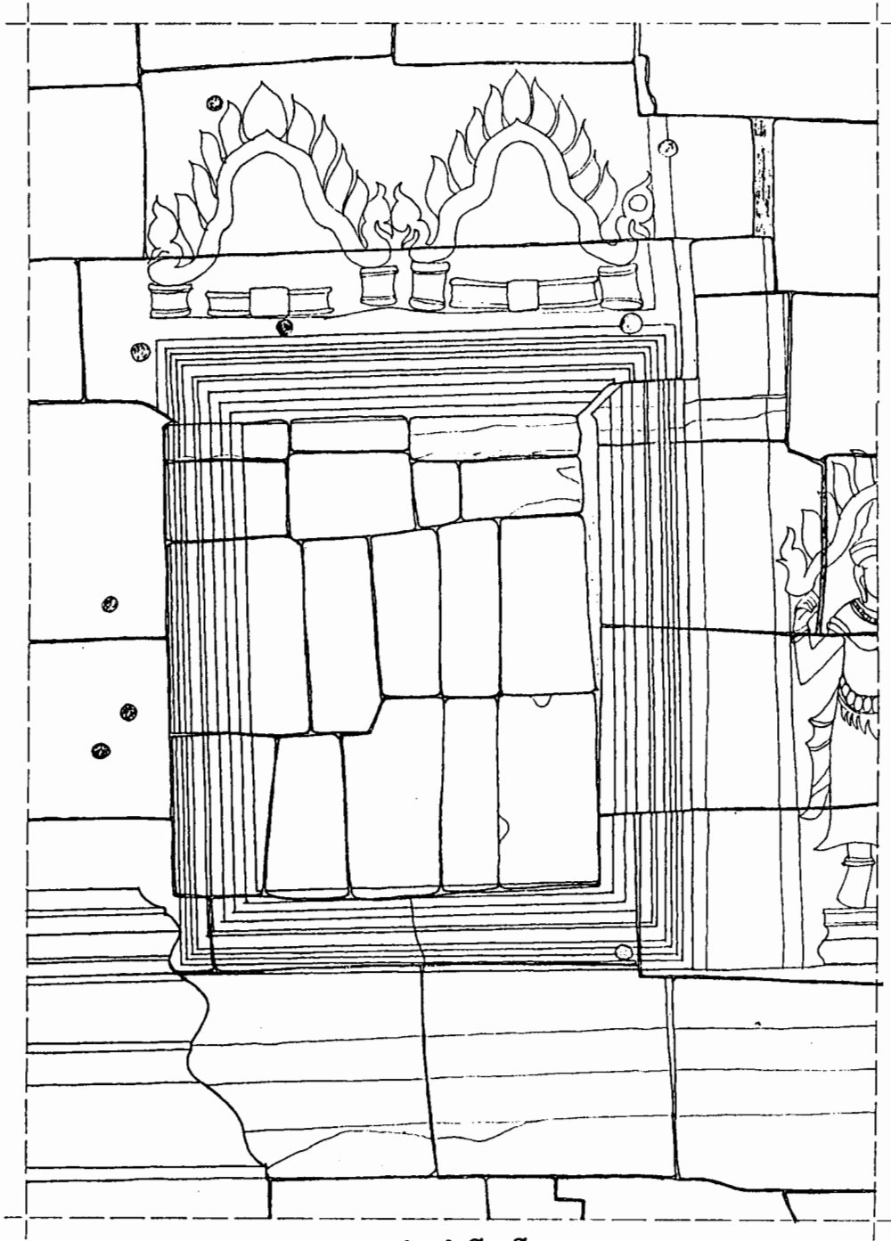
រូបភាពអំពីសំបើបពីខាងក្រៅ
