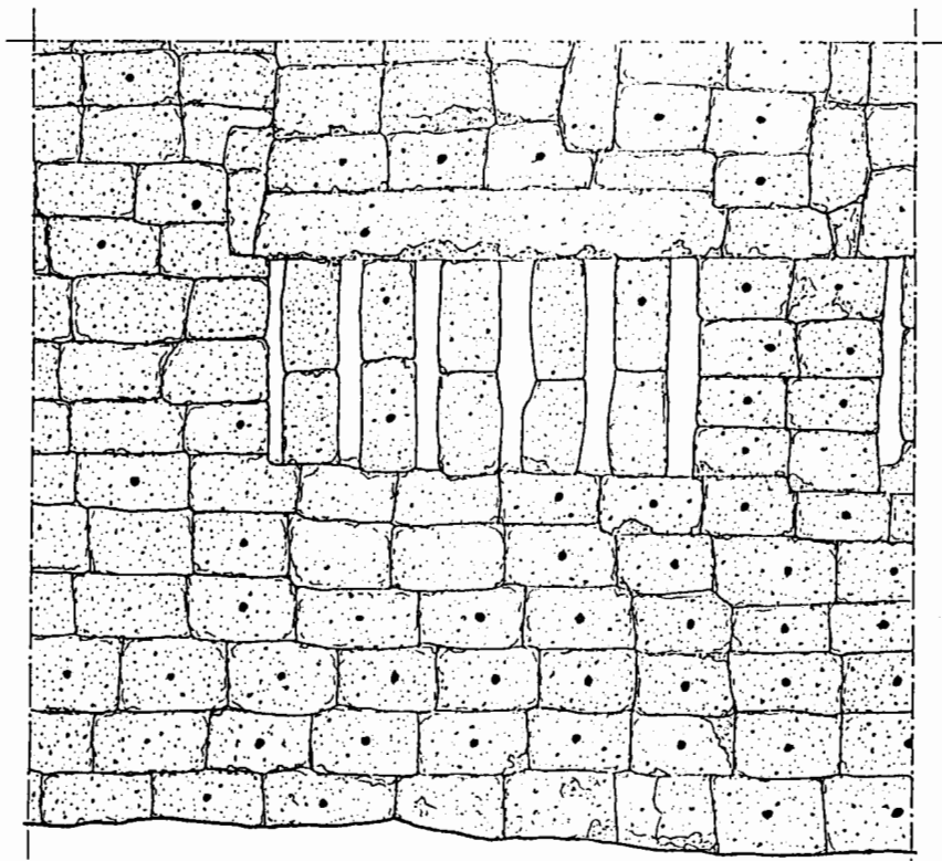
រូបភាពកំពស់មើលពីខាងក្រៅ
