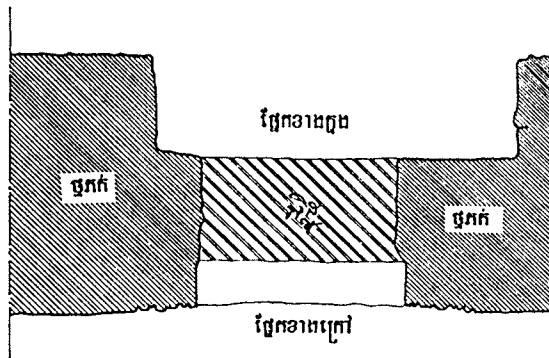
រូបគោតប្លង់នៃបង្គោល
