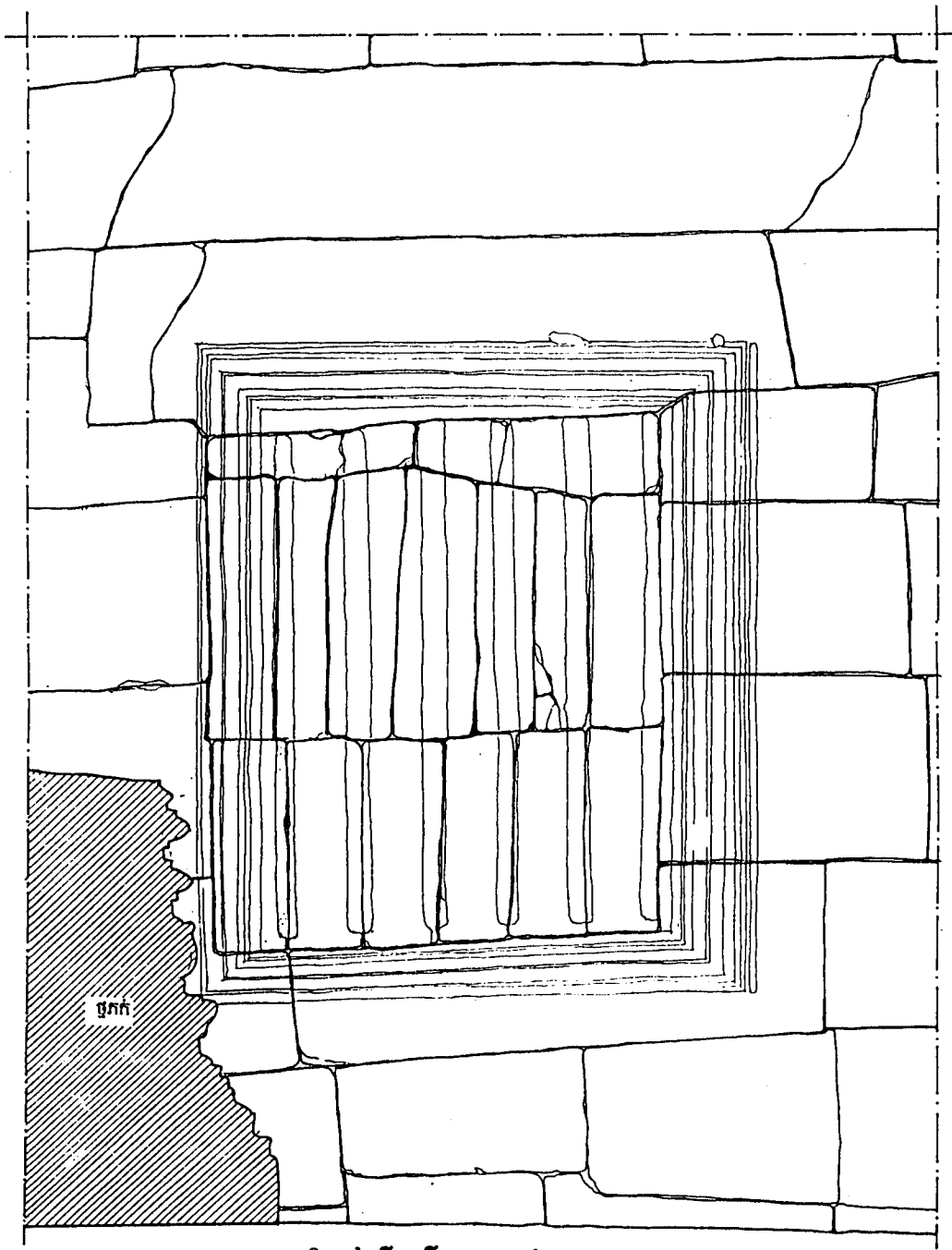
រូបគោតកំពស់មើលពីខាងក្រៅ ចារុតដ្ឋាន ១/១០
